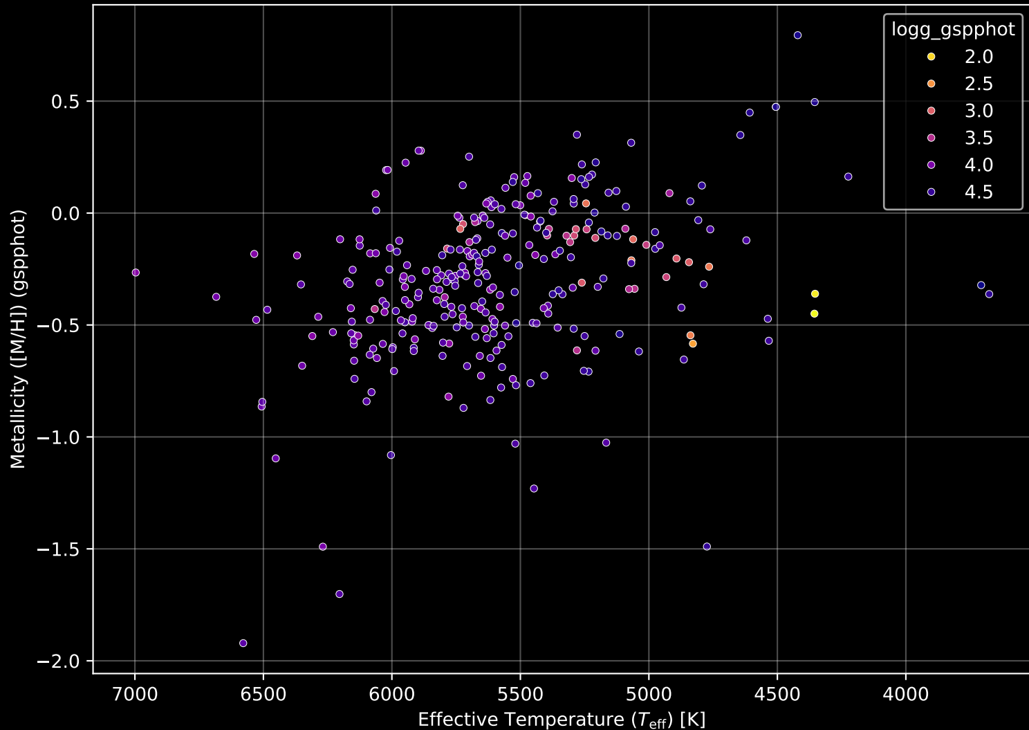
GALAH DR4 Field: [62] Stellar Population Parameters (n= 308)
