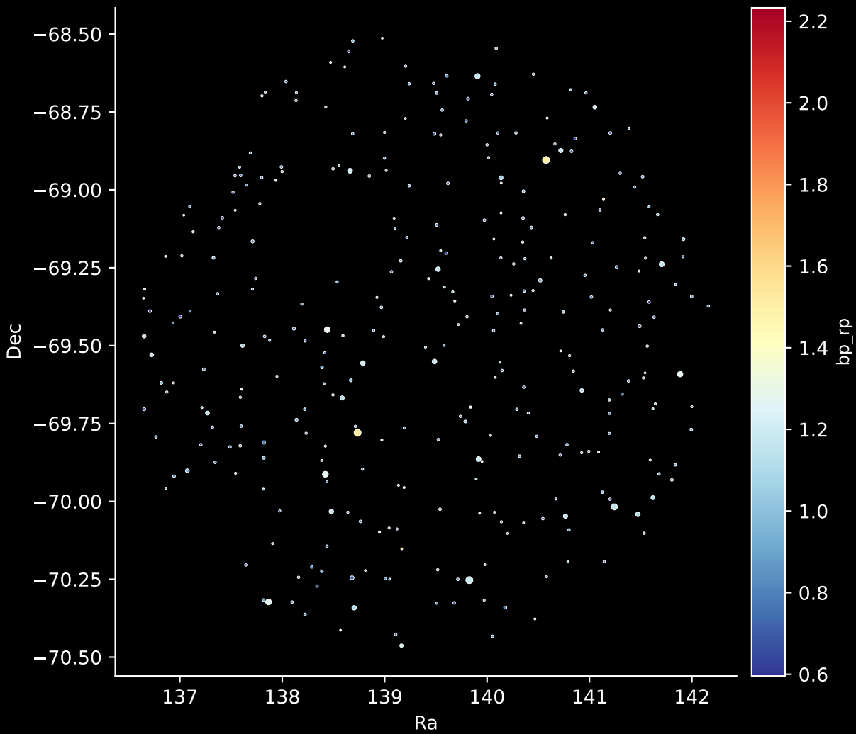
GALAH DR4 Field: [62] Stars: 308
